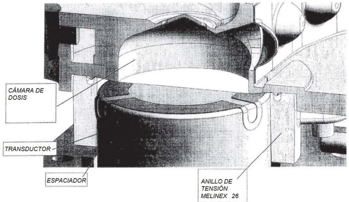
Figura 4: Mecanismo de Tensión Melinex que muestra un transductor, una cámara de dosis, un espaciador y un anillo de tensión melinex
