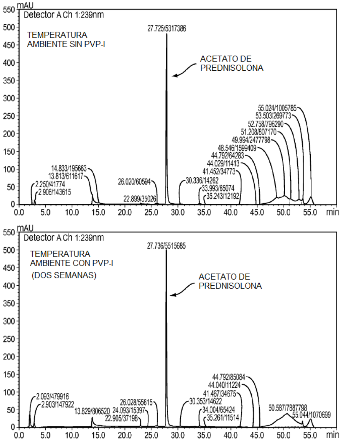
Cromatogramas HPLC-UV del acetato de prednisolona en PVP-I para dos semanas
