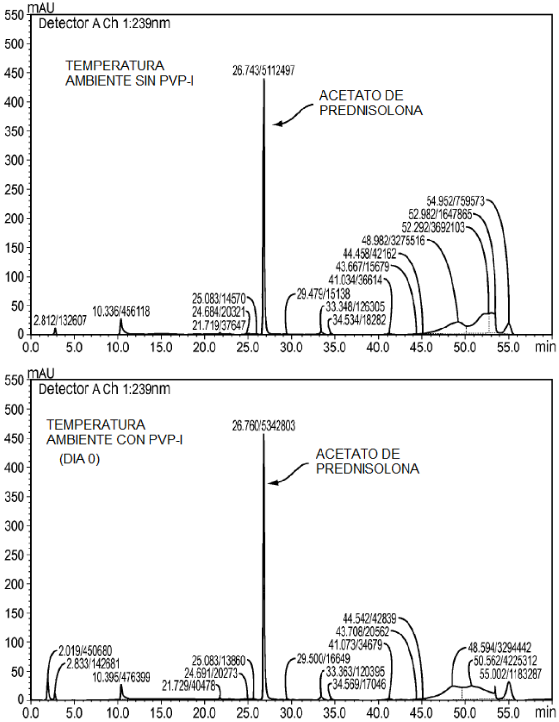
Cromatogramas HPLC-UV del acetato de prednisolona en PVP-I para el Día 0
