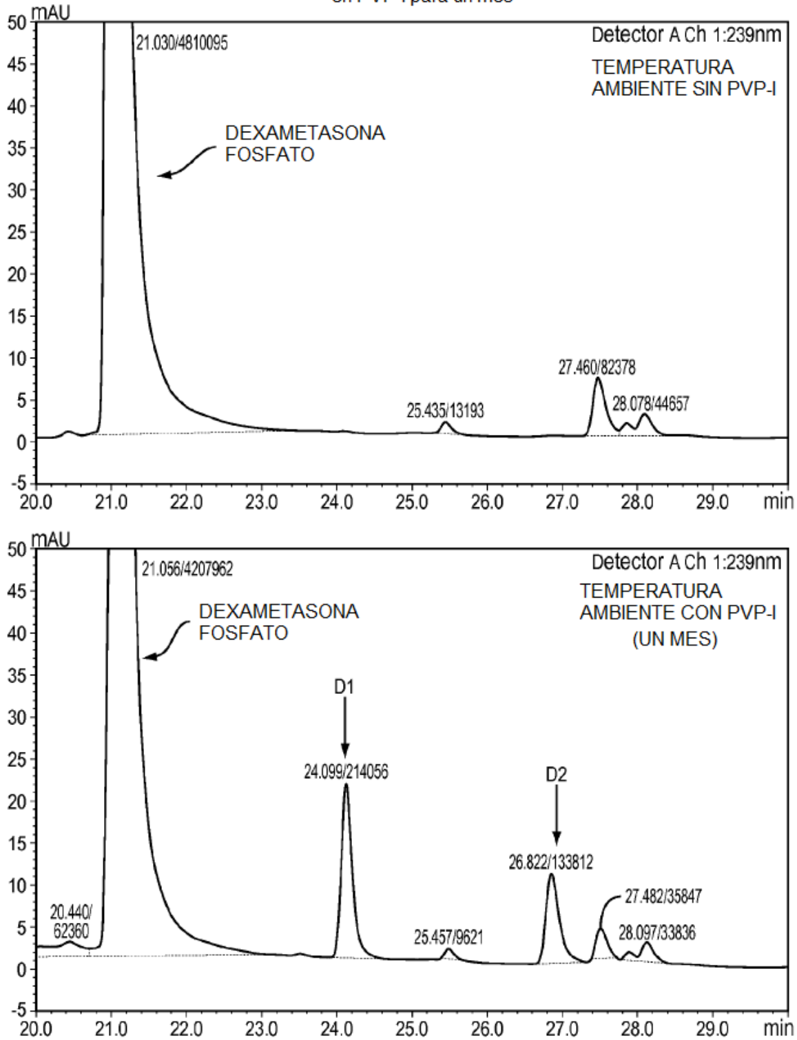
Cromatogramas HPLC-UV (expandidos) del fosfato de dexametasona sodio en PVP-I para un mes
