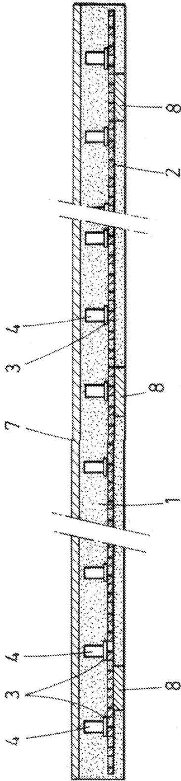
A-A FIG. 4
