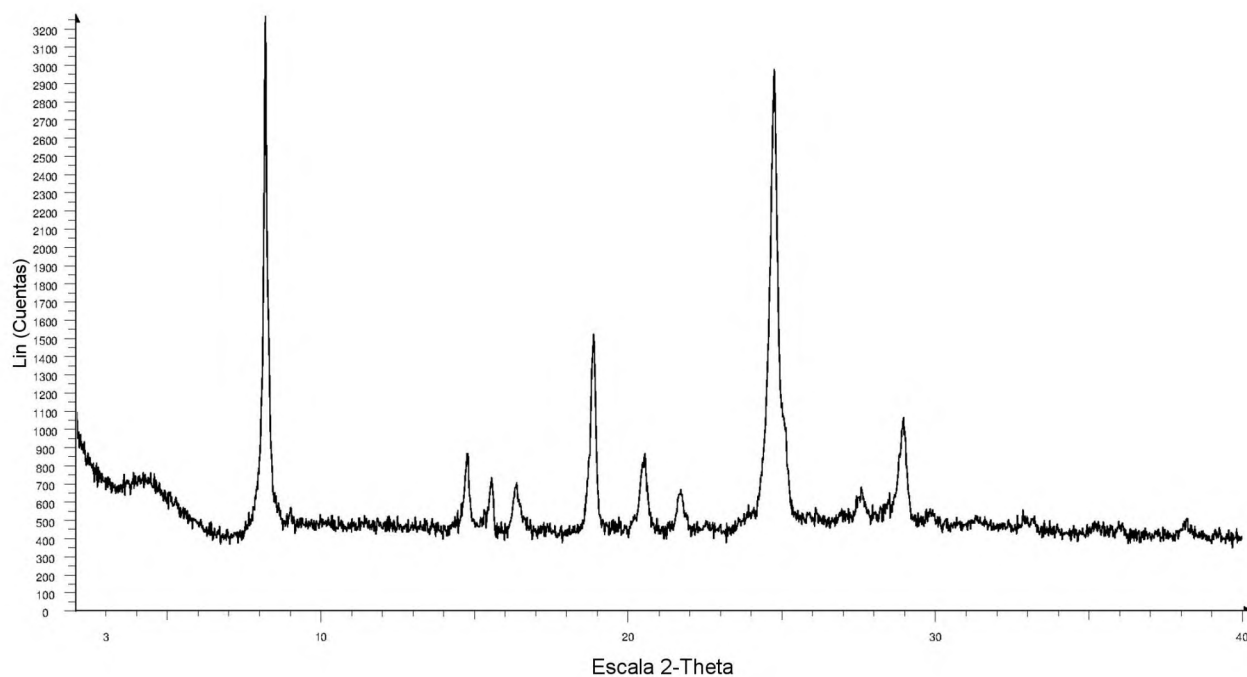
Figura M: Patrón de difracción de rayos X de polvo del cocrystal (1:1) del Compuesto A:ácido 6-hidroxi-2-naftoico, Forma C
