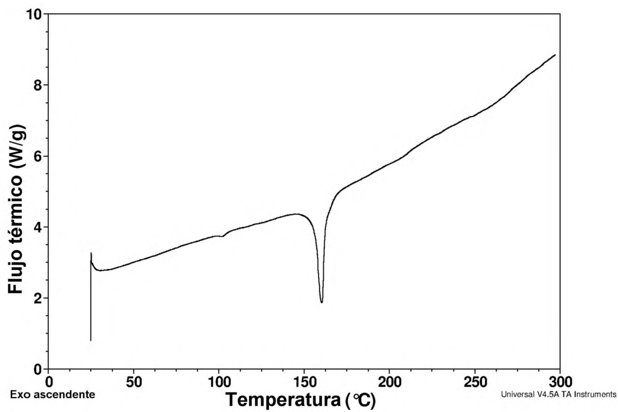
Figura N: Termograma de DSC del cocrystal (1:1) del Compuesto A:ácido 6-hidroxi-2-naftoico, Forma C
