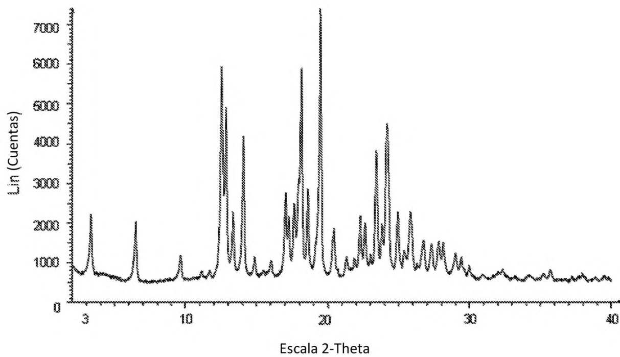
Figura C: Patrón de difracción de rayos X de polvo del cocrystal (1:1) del Compuesto A:ácido 6-hidroxi-2-naftoico, Forma A
