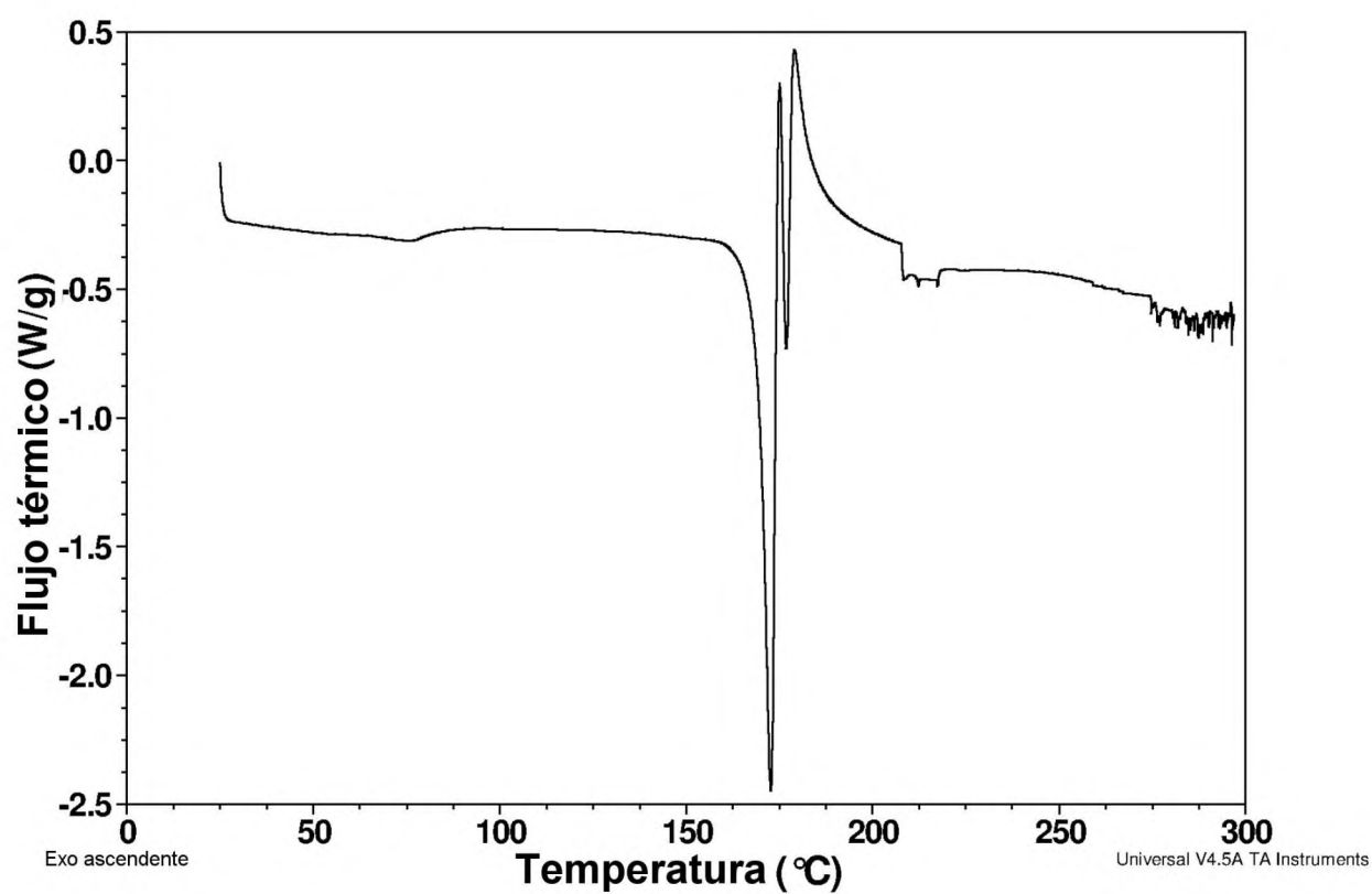
Figura L: Termograma de DSC del cocrystal (1:1) del Compuesto A:ácido 6-hidroxi-2-naftoico, Forma B
