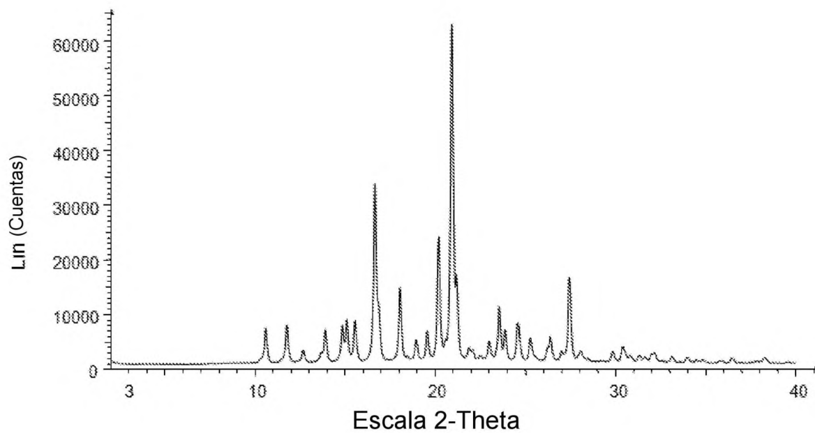
Figura A: Patrón de difracción de rayos X de polvo del Compuesto A, Forma A
