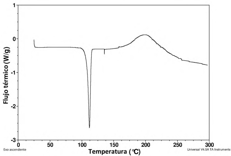
Figura B: Termograma de DSC del Compuesto A, Forma A
