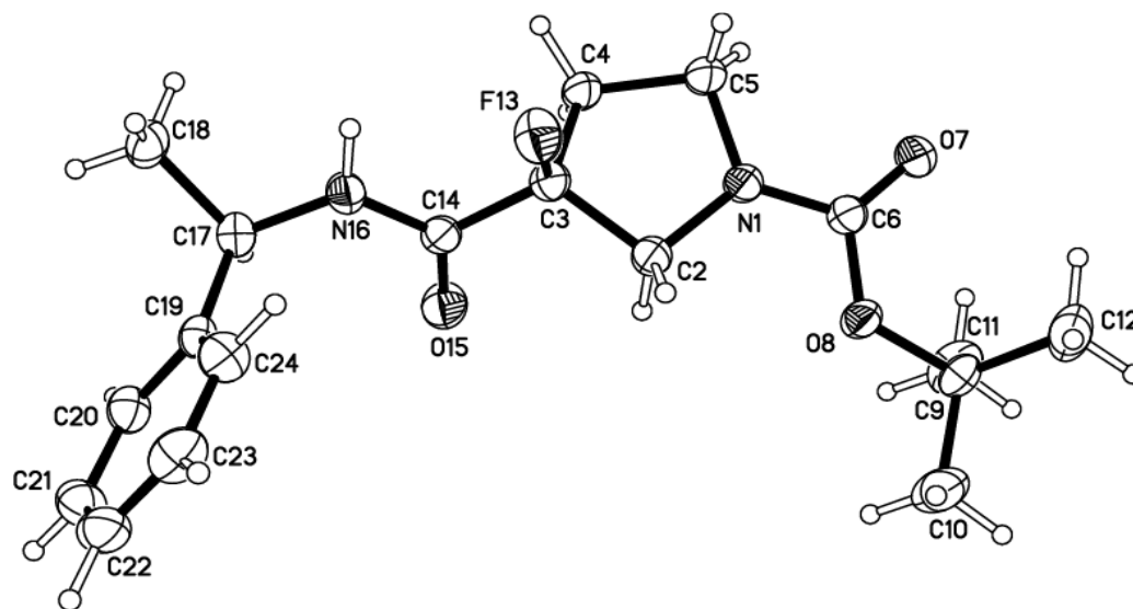
Figura 1. La estructura cristalina por rayos X del compuesto (XVIII)
