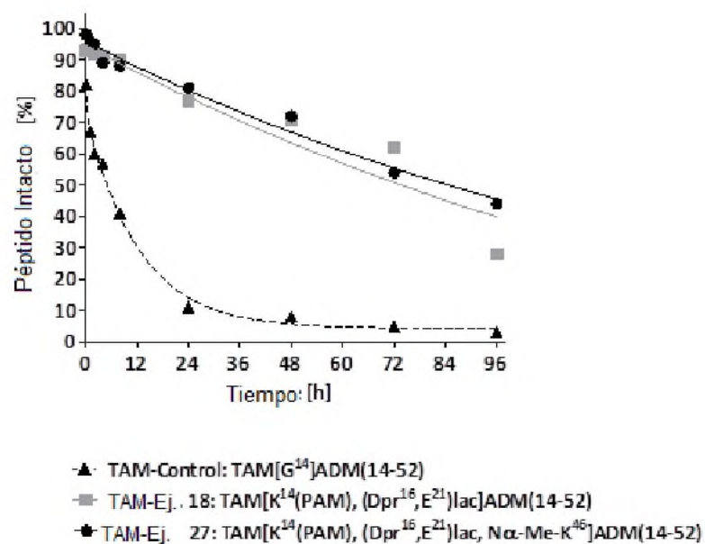
Fig. 3: Estabilidad de péptidos en plasma.
