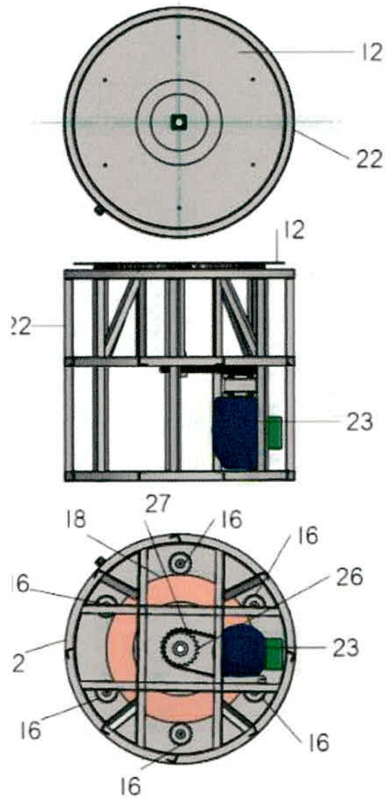
Ilustración 6. Disposición del motor en el Chasis
