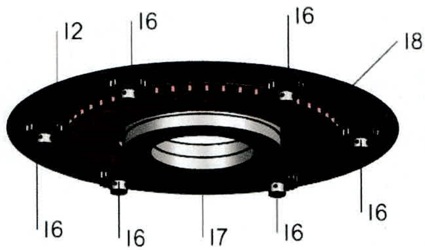
Ilustración 9. Disco inferior con cremallera con piñones satélites.
