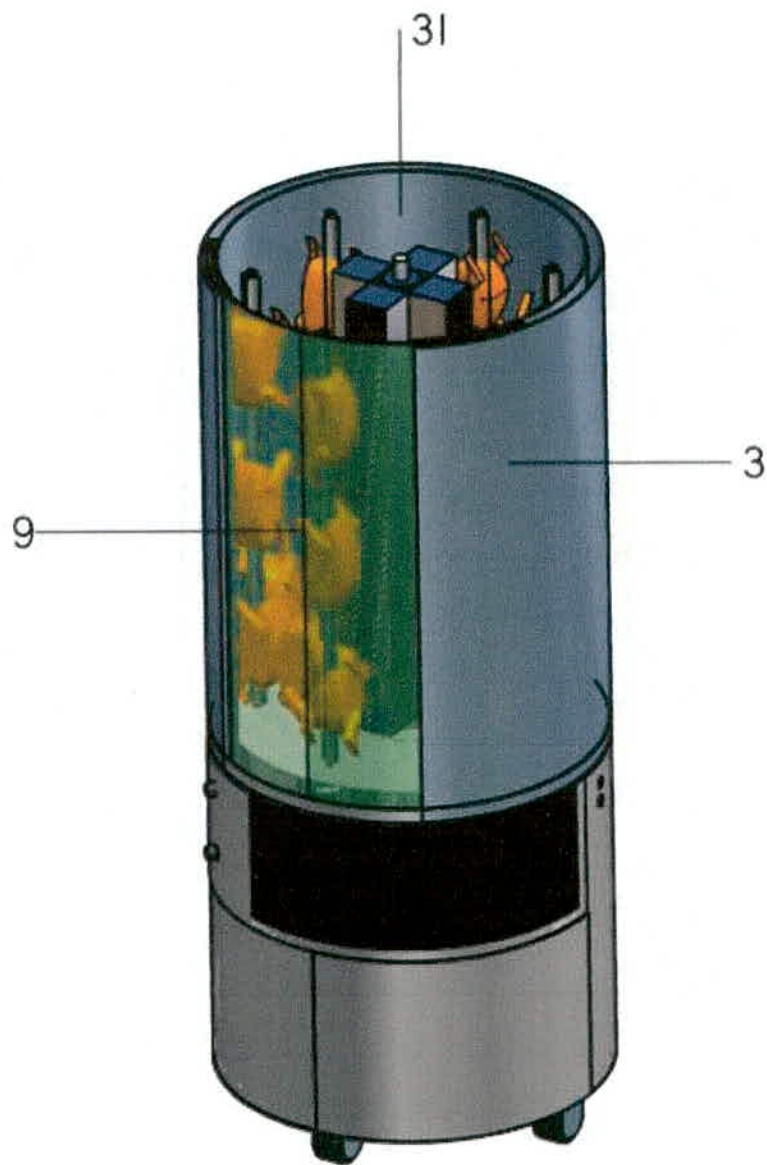
Ilustración 10. Cámara de calentamiento (10)
