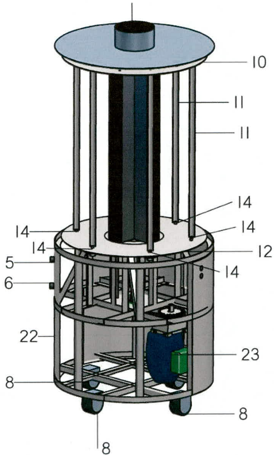
Ilustración 8. Ensamble chasis con sistema de rotación.
