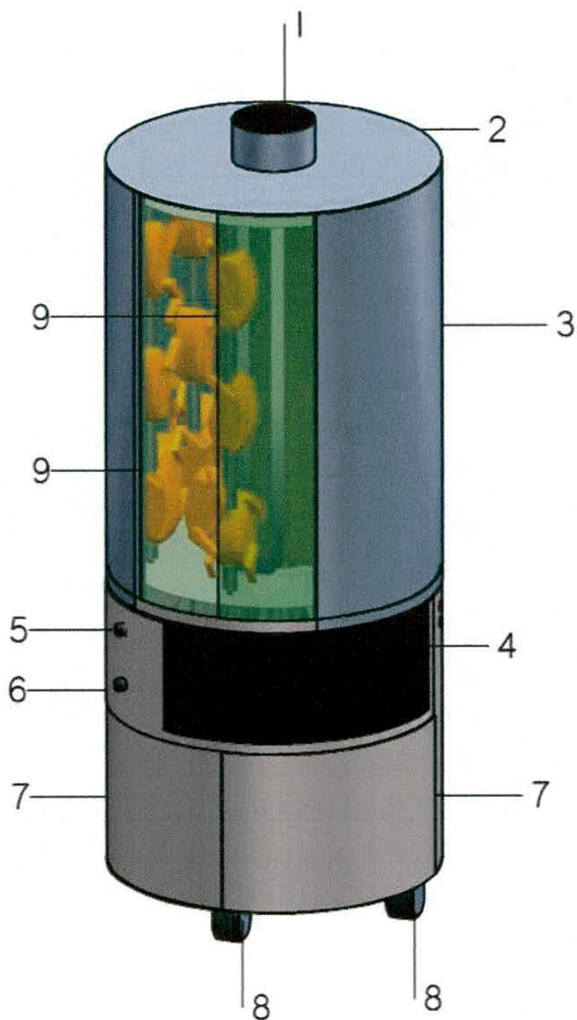
Ilustración 1. Estructura externa Horno vertical circular para asado de pollo.
