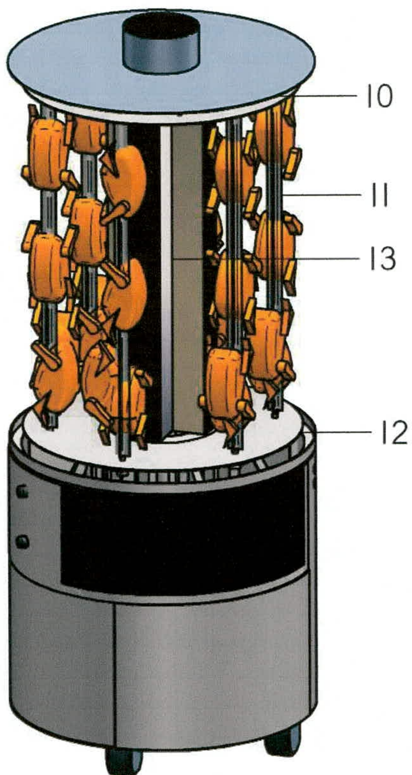
Ilustración 2. Disposición de los pollos para asar dentro del Horno vertical circular para asado de pollo
