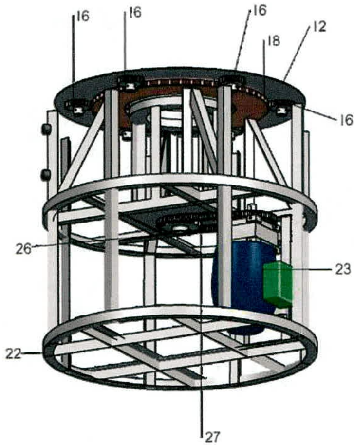
Ilustración 7. Chasis Horno
