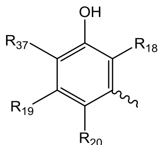
Fórmula (IVb)
