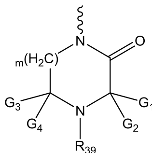
Fórmula (IIa)
