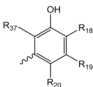
Fórmula (IVa)
