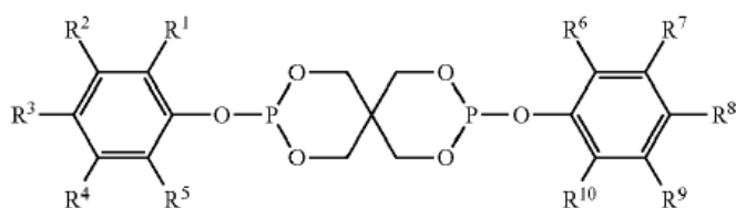
Fórmula (V)
