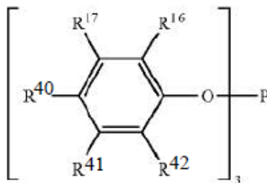
Fórmula (VI)
