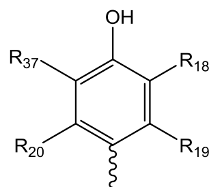
Fórmula (IVc)
