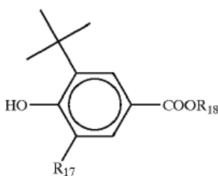
Fórmula (III)
