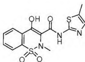
Meloxicam
