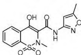
Isoxicam
