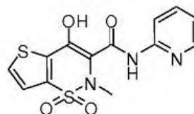
Tenoxicam
