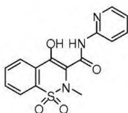
Piroxicam
