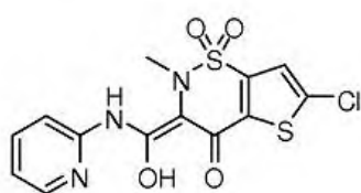
Lornoxicam
