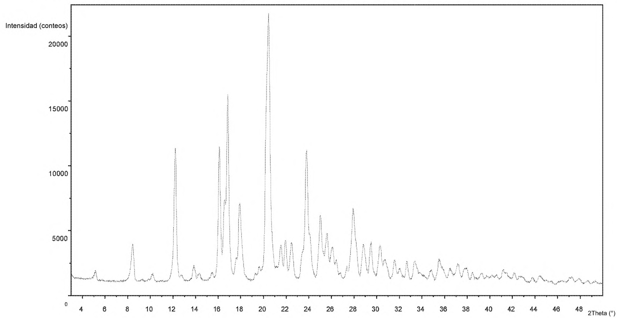
Figura 1: XRD en polvo. Patrones de difracción de la Forma B de ARN-509.
