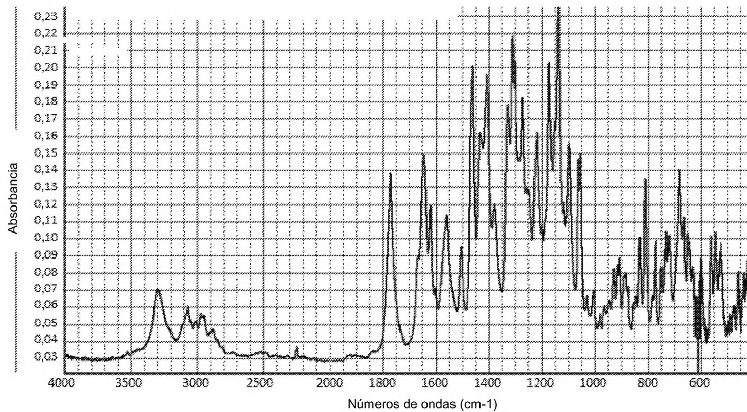
Figura 2: Espectrometría Irared (microATR) de la Forma B de ARN-509.
