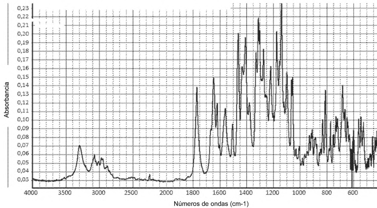
Figura 2: Espectometría Irared (microATR) de la Forma B de ARN-509.
