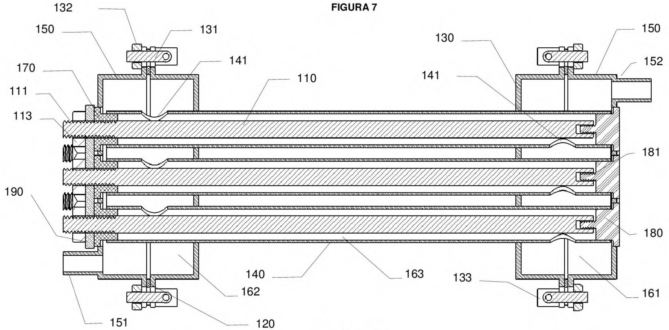
SECCIÓN A-A
