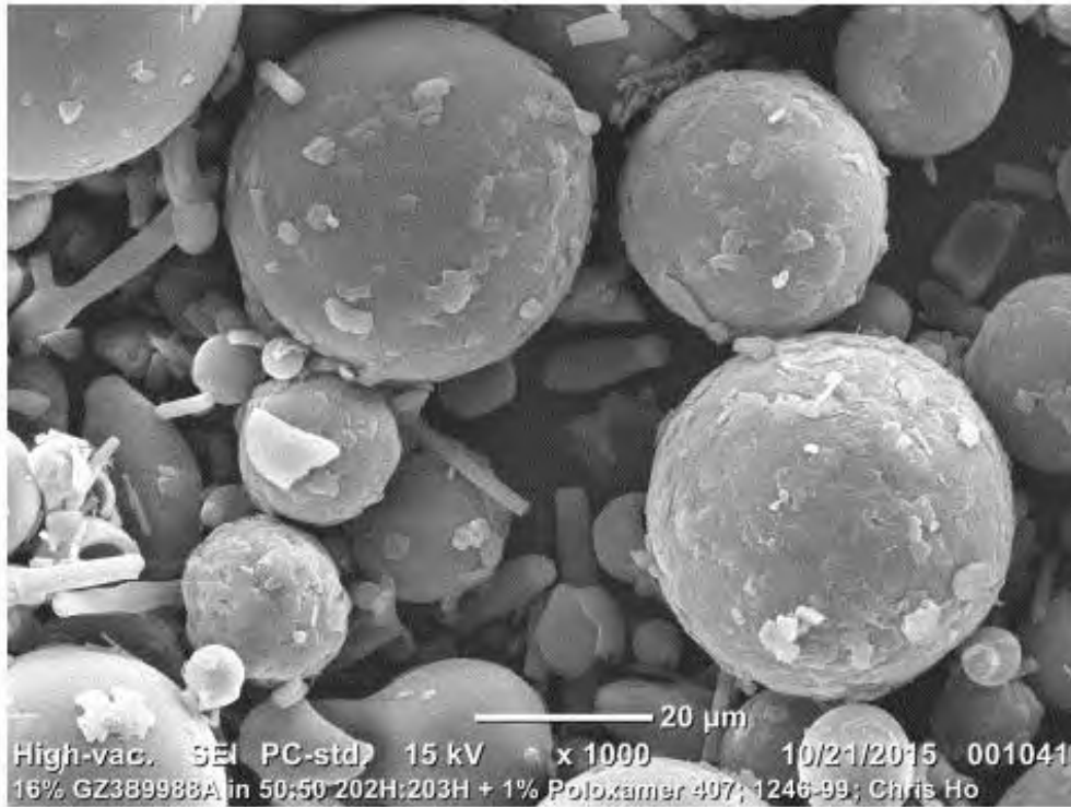
Figura 23: Vista de microscopía electrónica de barrido (SEM) de Microesferas de 16 % de API/1:1 de R202H:R203H/31,25 mg de Poloxámero 407, Secadas por pulverización (1000X)
