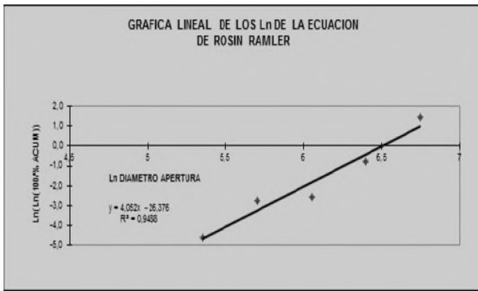
Figura 11. Muestra la gráfica lineal de los Ln de la ecuación de Rosin-Ramler para el café Italiano molido
