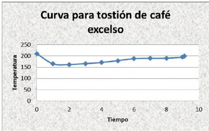
Figura 2. Muestra la curva de tostión para 150 gramos de café excelso
