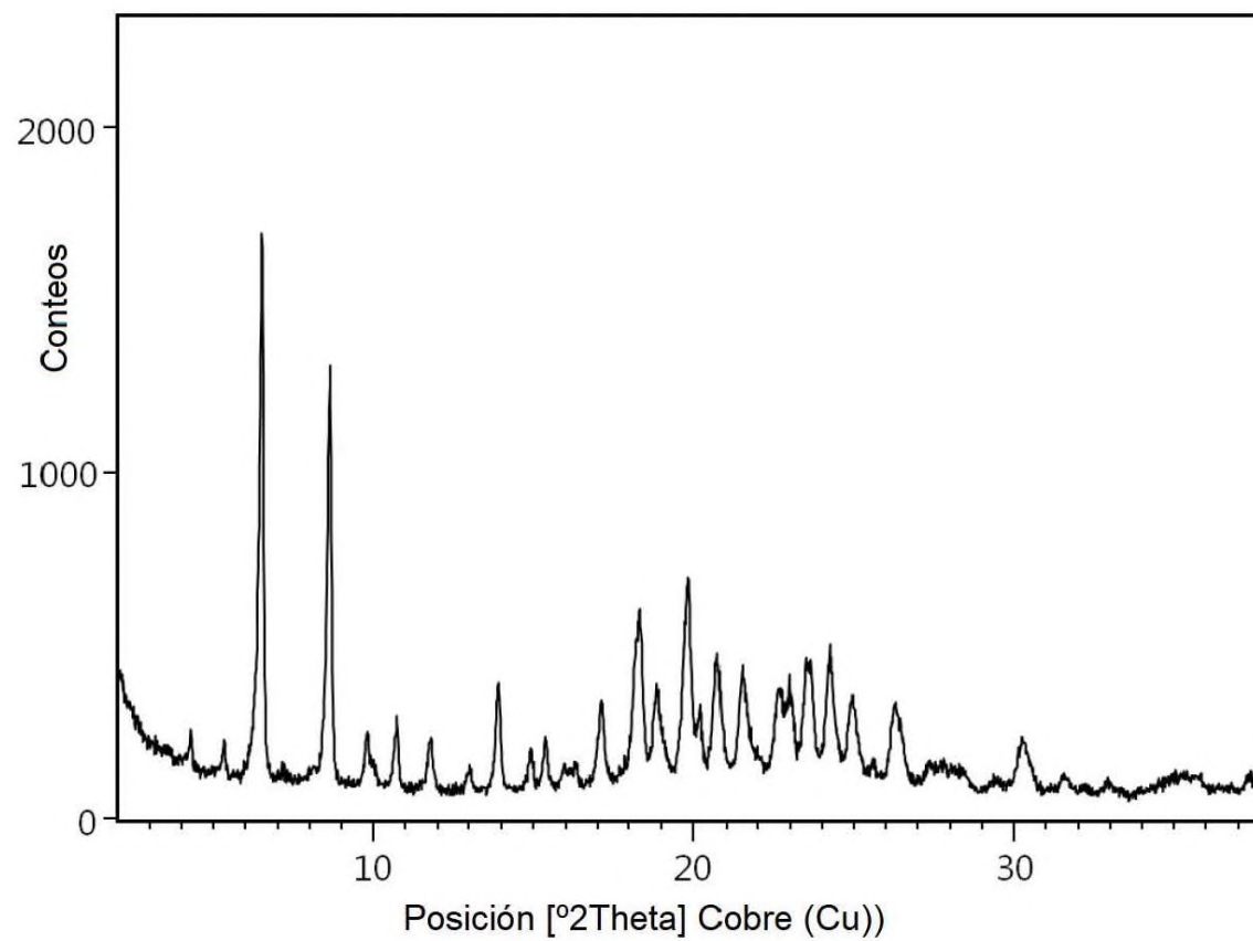
Figura 1: difractograma de rayos X del compuesto de la fórmula (I) en forma cristalina de la modificación I
