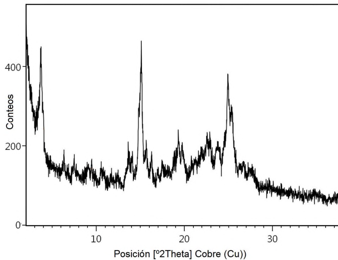
Figura 2: difractograma de rayos X del compuesto de la fórmula (I) en forma cristalina de la modificación II
