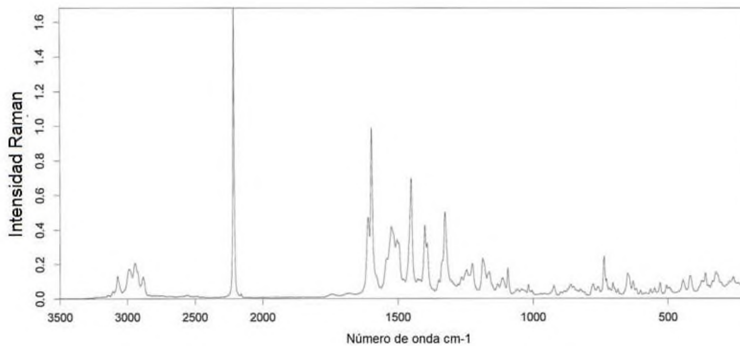
Figura 9: Espectro Raman del compuesto de la fórmula (I) en forma cristalina de la modificación IV
