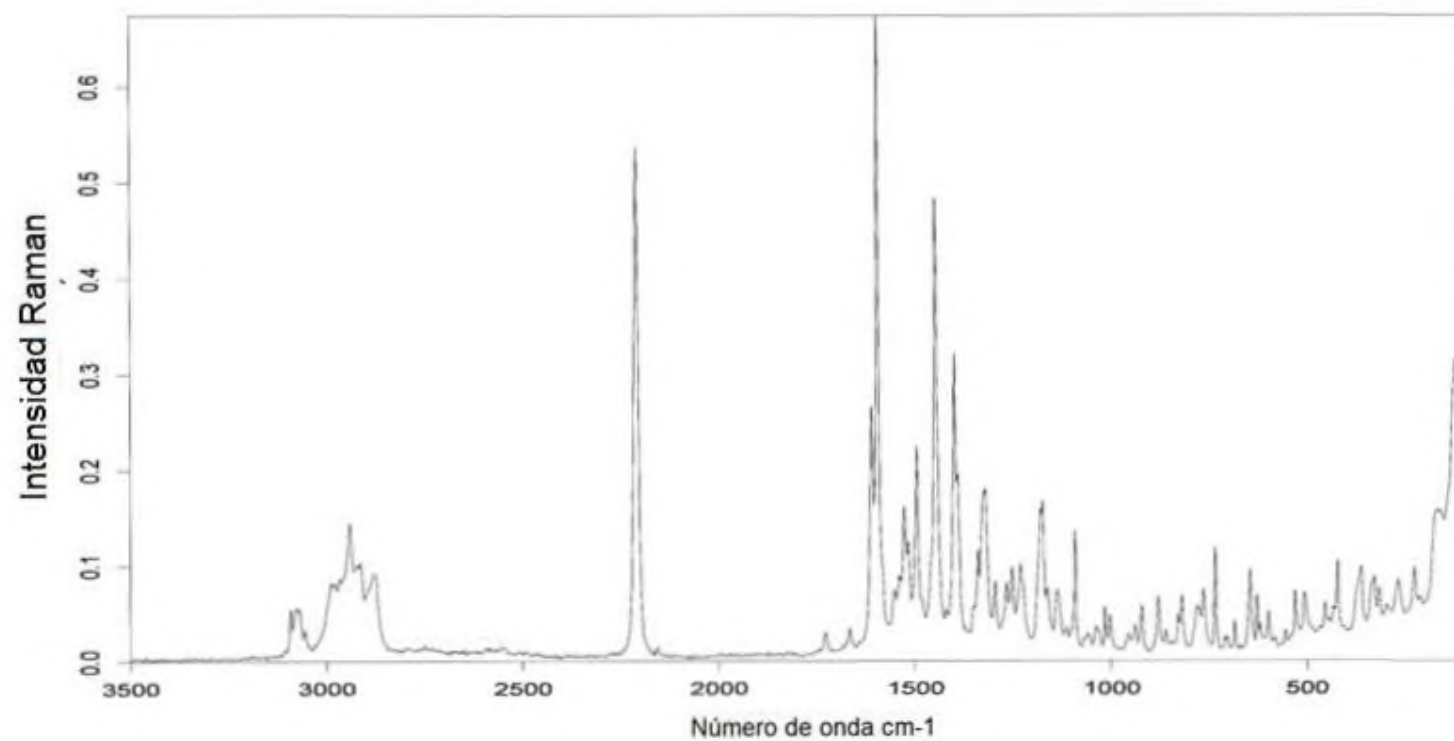
Figura 10: Espectro Raman del compuesto de la fórmula (I) en forma cristalina del solvato de isopropanol
