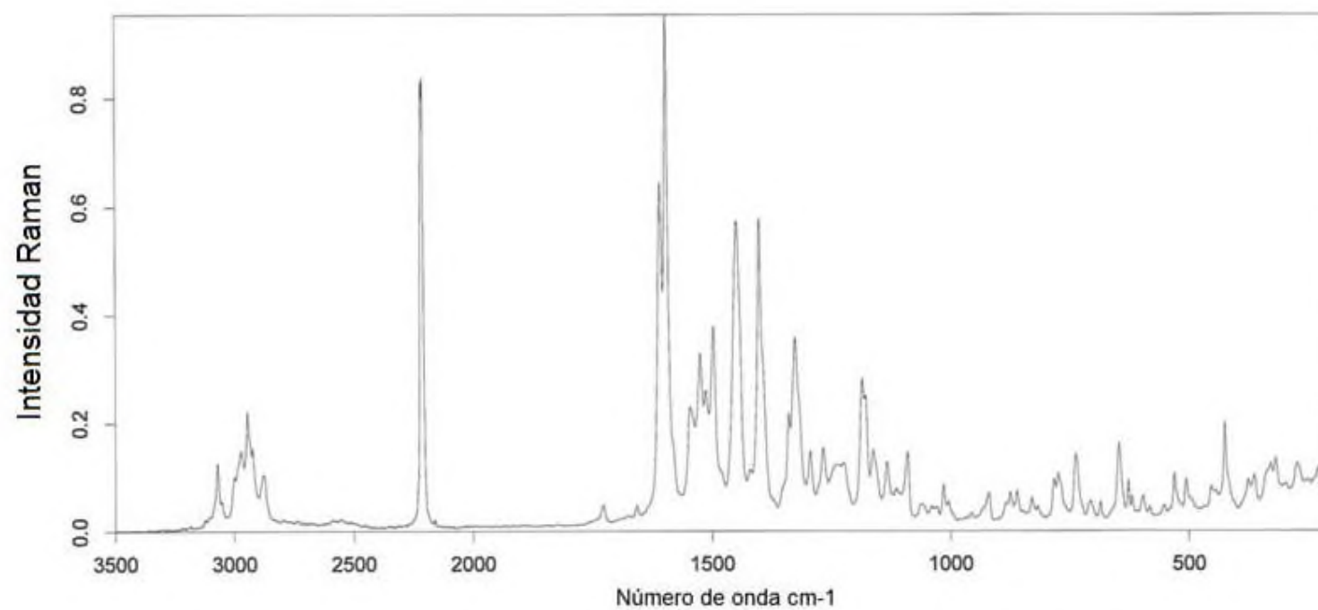
Figura 8: Espectro Raman del compuesto de la fórmula (I) en forma cristalina de la modificación III
