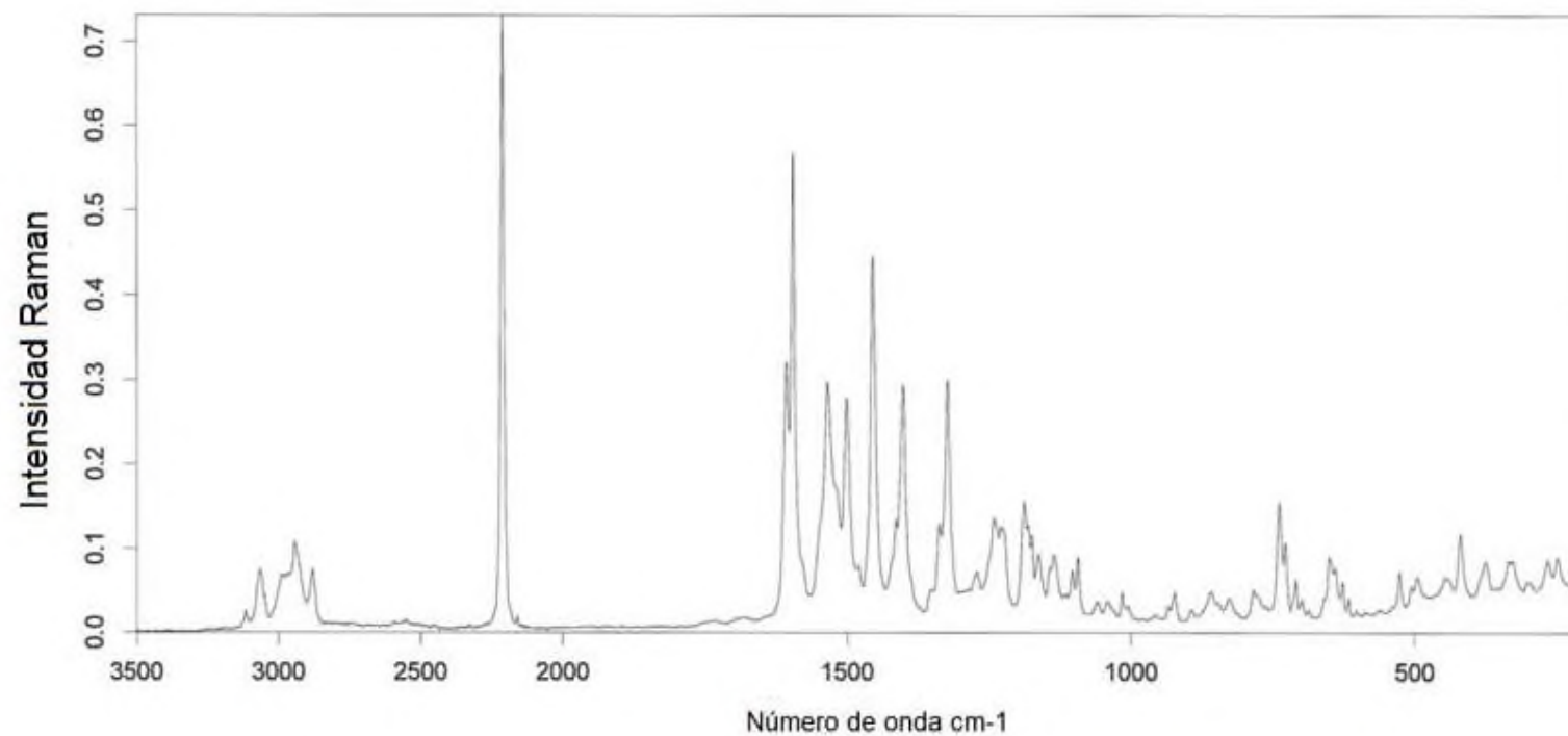
Figura 7: Espectro Raman del compuesto de la fórmula (I) en forma cristalina de la modificación II
