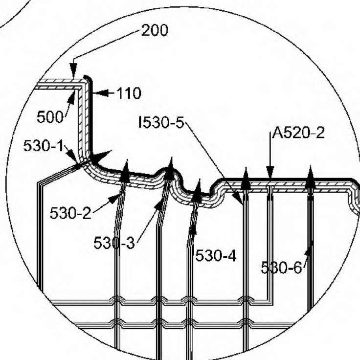
DETALLE B
