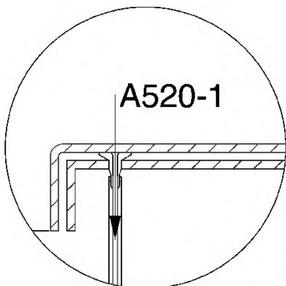
DETALLE A
