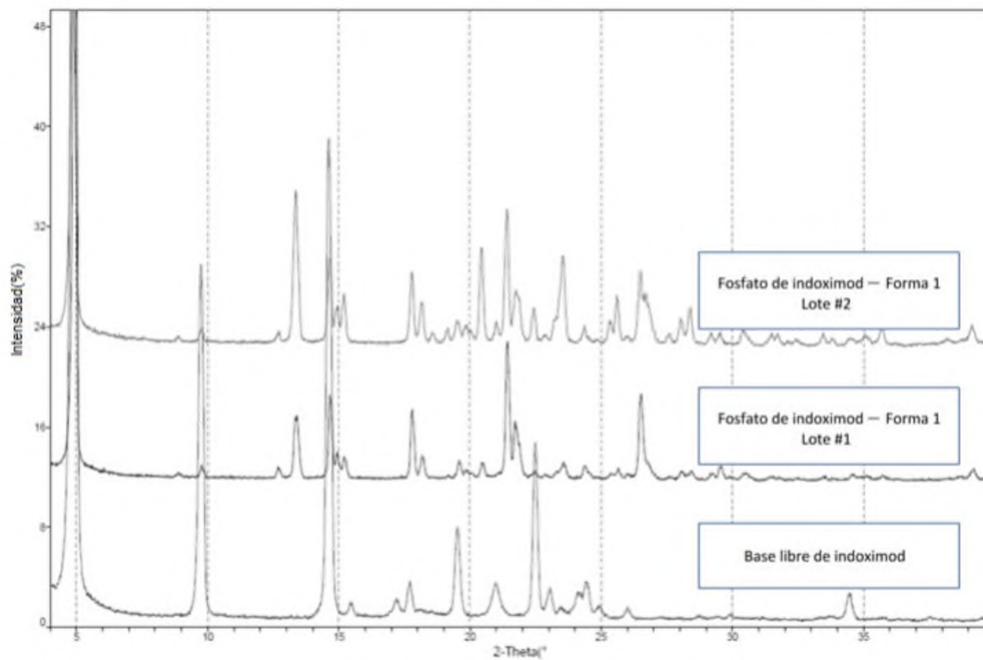
Figura 3: XRPD de indoximod y fosfato de indoximod
