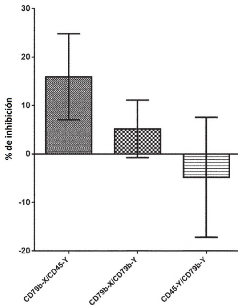
Figura 1 pAkt S473 en células B
