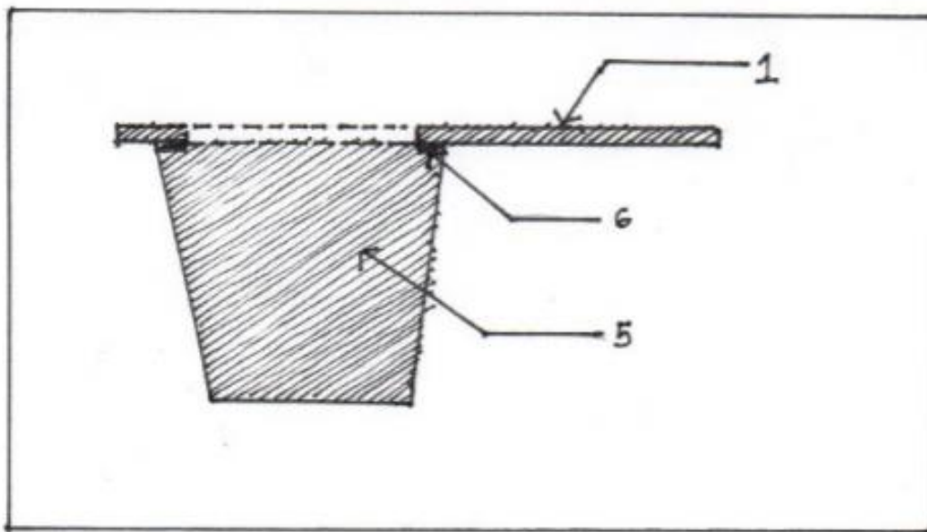
FIGURA No 2 - VISTA LATERAL
