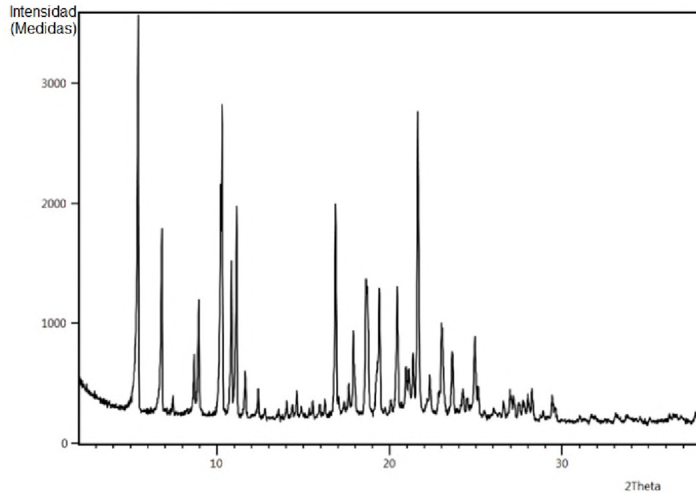
Fig. 2: Difractograma de rayos-X.
