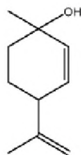
mentadienol
