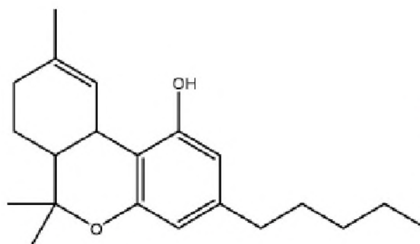
delta-9-tetrahidrocannabinol
