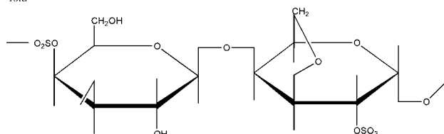
Iota
