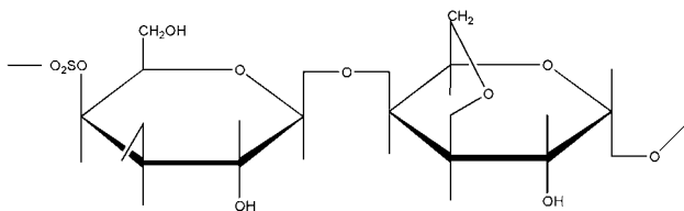
Kappa
