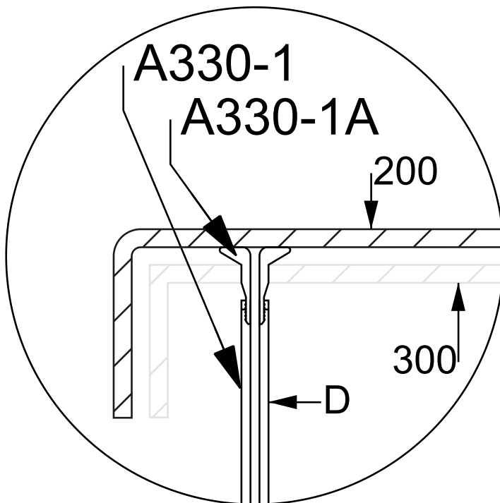
DETALLE A
