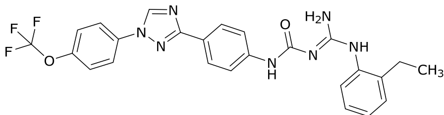
(1E)-1-[Amino-(2-metilanilino)metileno]-3-[4-[1-[4-(trifluorometoxi)fenil]-1H-1,2,4-triazol-3-il]fenil]urea (F5)
