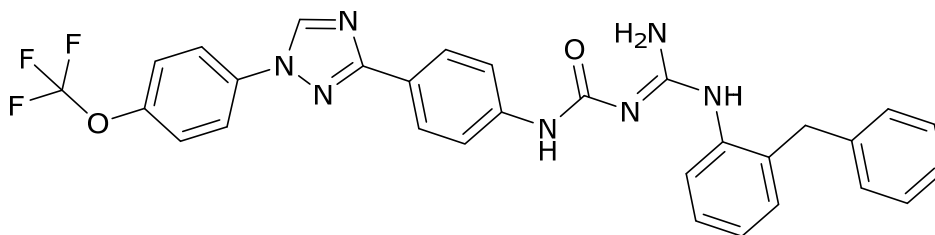
(1E)-1-[Amino-(2-tilanilino)metileno]-3-[4-[1-[4-(trifluorometoxi)fenil]-1H-1,2,4-triazol-3-il]fenil]urea (F3)
