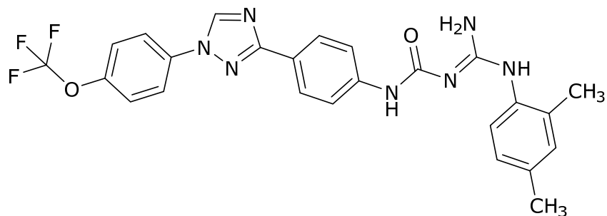
10 (1E)-1-[Amino-(4-metoksi-2-metil-anilino)metileno]-3-[4-[1-[4-(trifluorometoxi)fenil]-1H-1,2,4-triazol-3-il]fenil]urea (F9)
