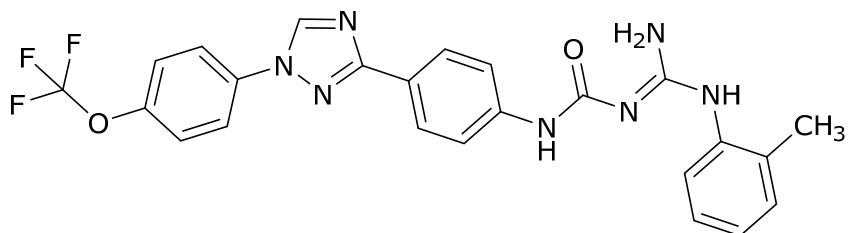
(1E)-1-[Amino-(2-metilanilino)metileno]-3-[4-[1-[4-(trifluorometoxi)fenil]-1H-1,2,4-triazol-3-il]fenil]urea (F5)
