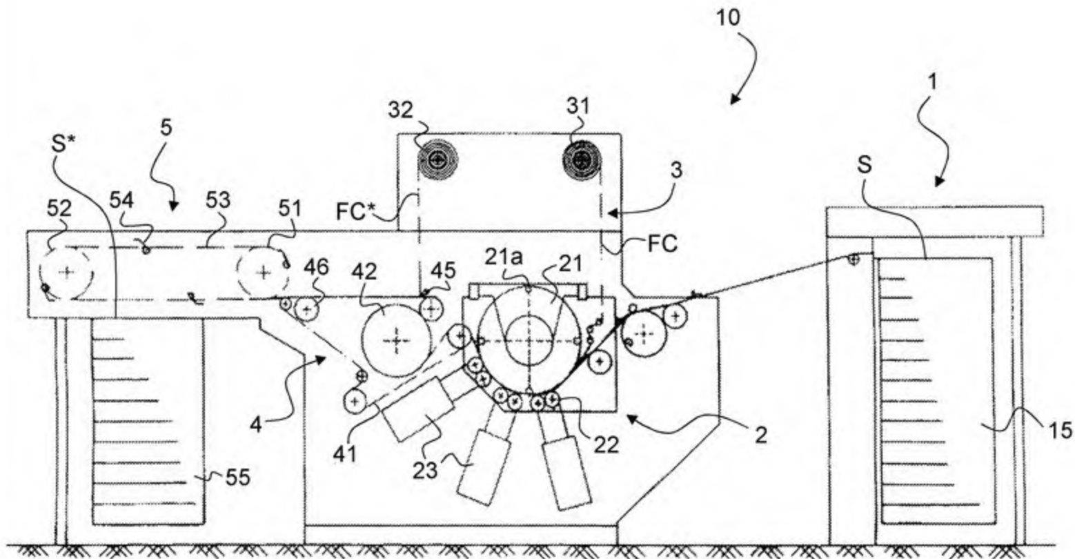
Fig. 1 (TÉCNICA ANTERIOR)
