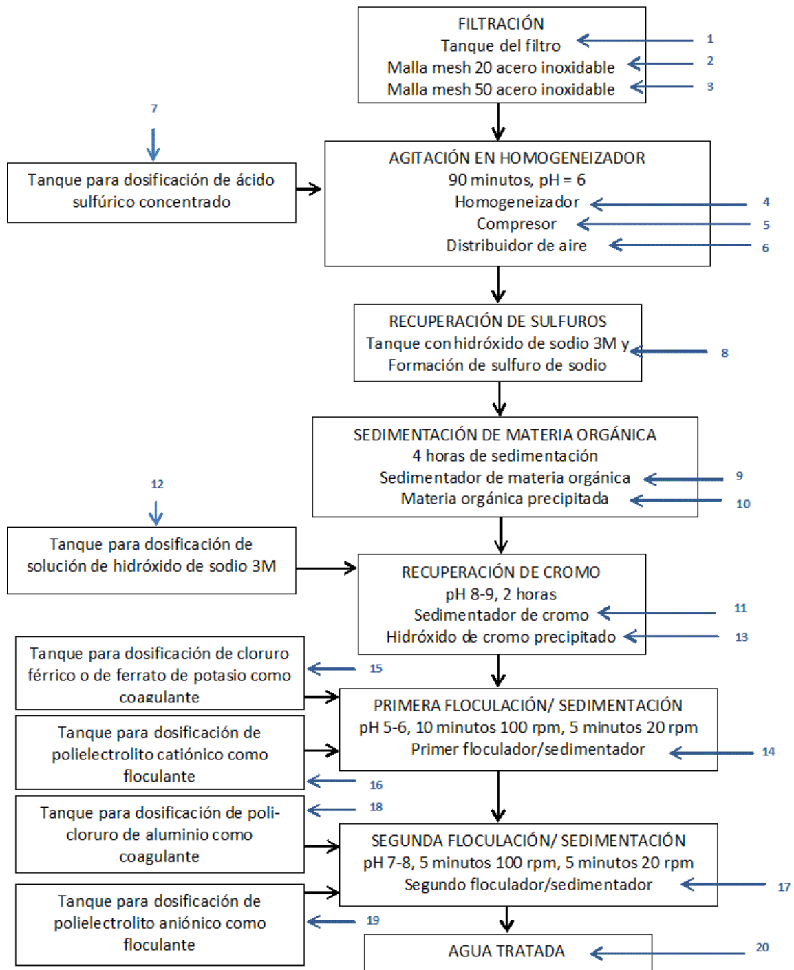
Figura 2. Diagrama de flujo del proceso de tratamiento de aguas residuales de curtiembres con recuperación de sulfuros, cromo y materia orgánica
