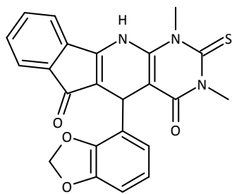
(Compuesto VIII).
