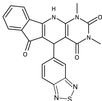
(Compuesto XI).
