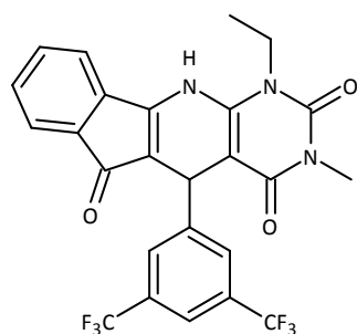
(Compuesto VI).
