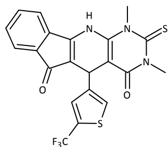
(Compuesto II).
