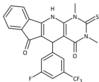
(Compuesto III).
