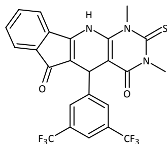
(Compuesto V).
