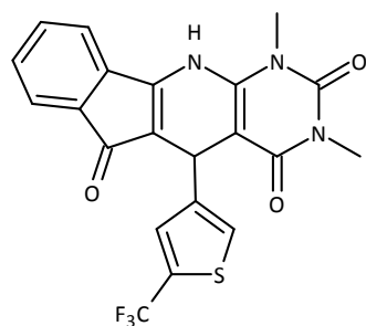
(Compuesto I).
