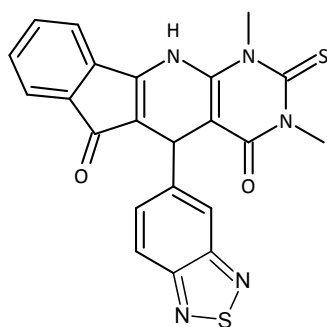
(Compuesto XII).
