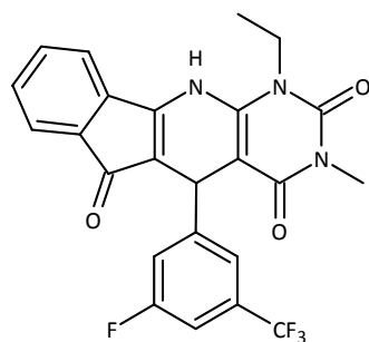
(Compuesto IV).
