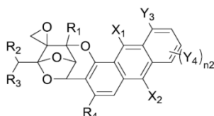
Fórmula Ib
