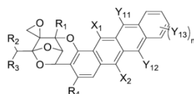
Fórmula If
