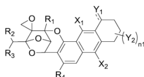
Fórmula Ia
