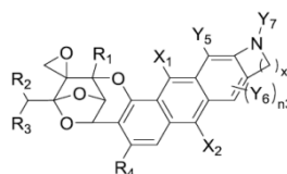
Fórmula Ic
