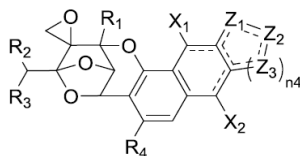
Fórmula Id
