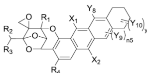
Fórmula Ie
