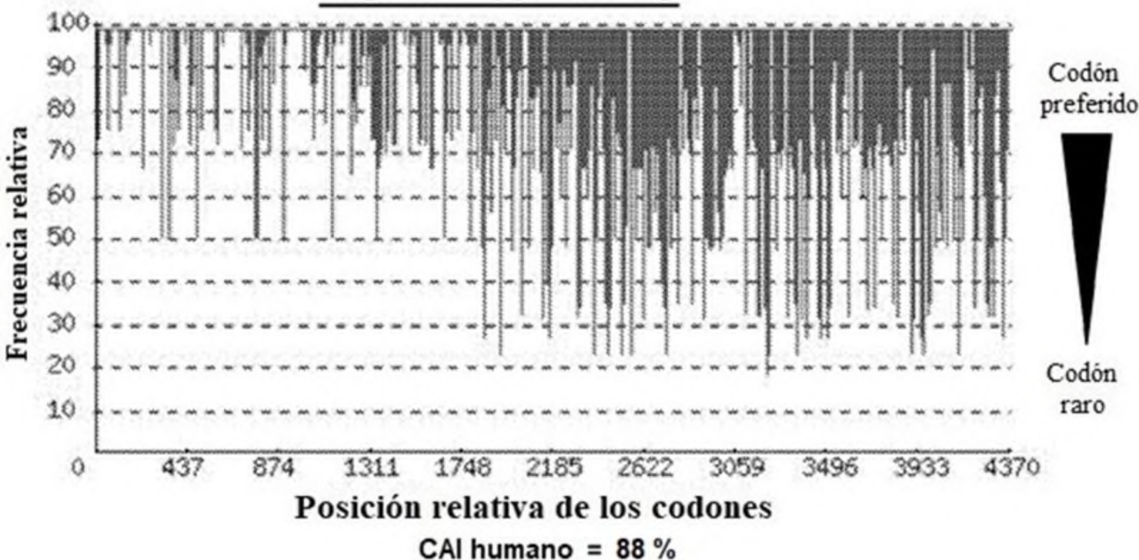
FIG. 2I – coFVIII-25
