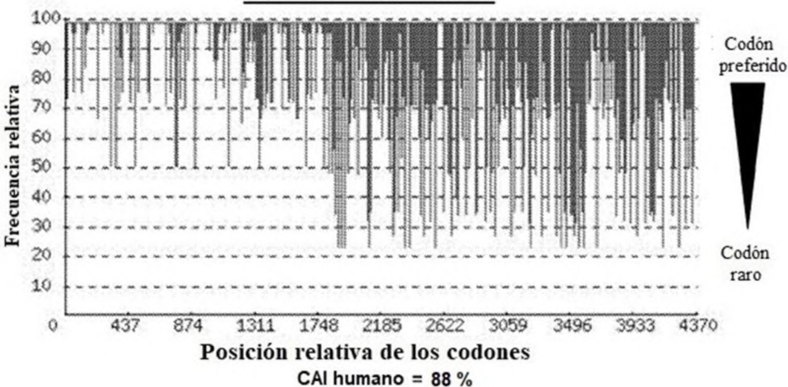
FIG. 2J – coFVIII-26
