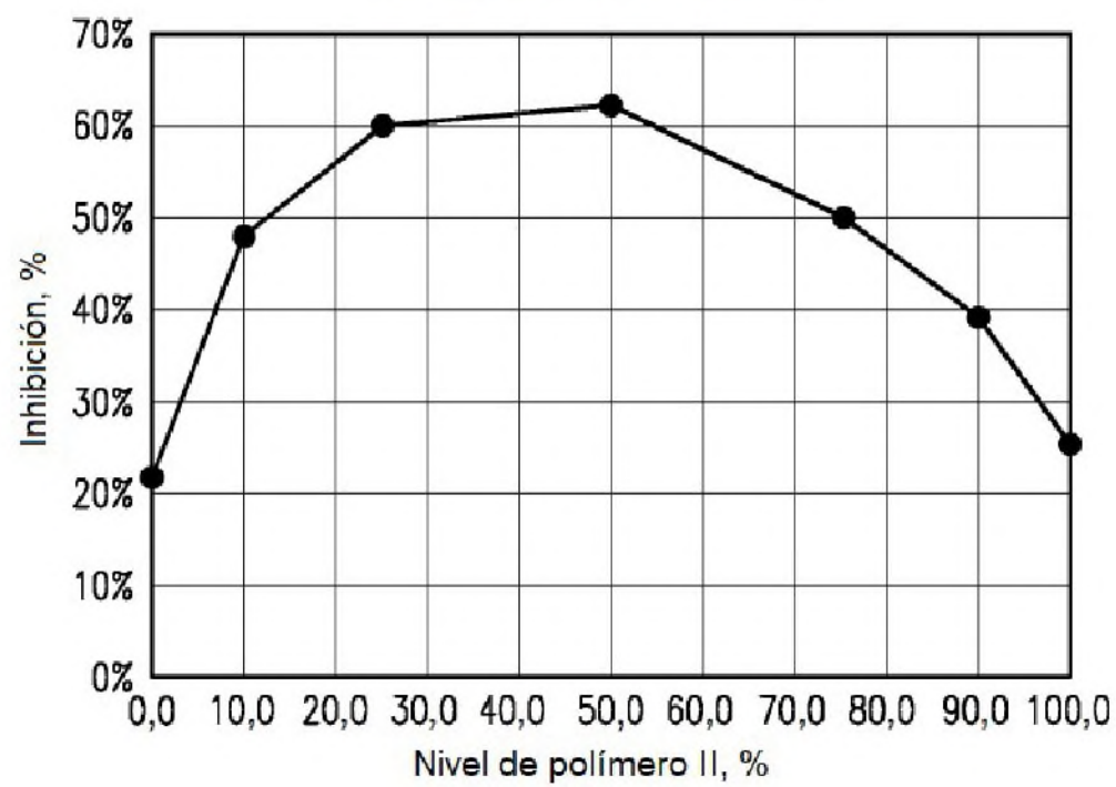
Desempeño de inhibición de varias mezclas de Polímero I y II 125 ppm de nivel de tratamiento
