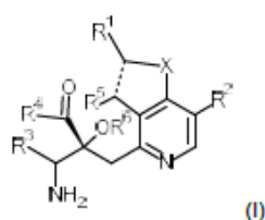
Fórmula Química 2
