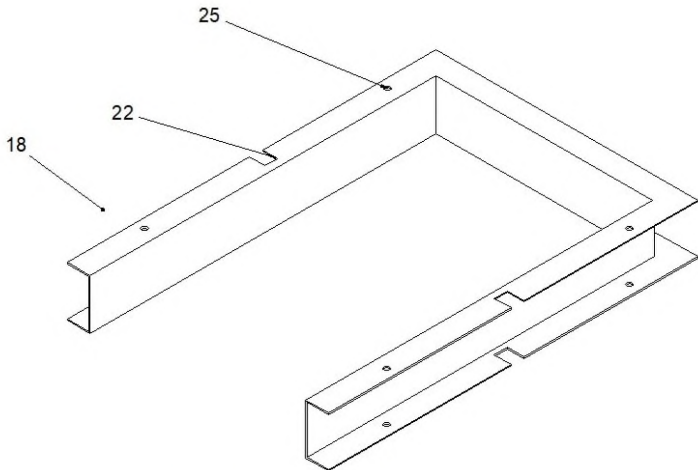
Figura 4. Vista en perspectiva de miembro espaciador
