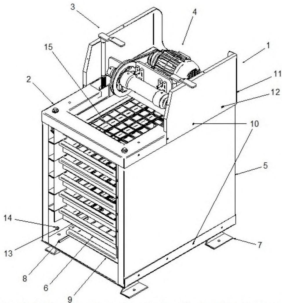
Figura 1. Vista en perspectiva de la máquina tamizadora
