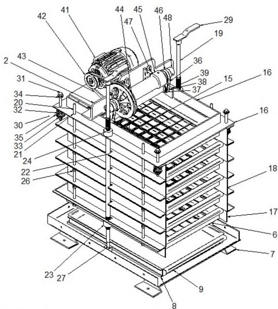
Figura 2. Vista en perspectiva de partes internas de la máquina tamizadora
