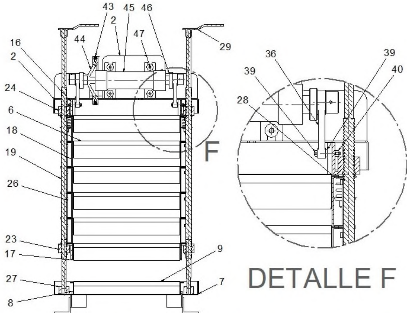
Figura 3. Corte en sección transversal frontal de la máquina tamizadora
