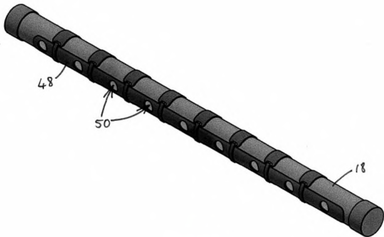
FIGURA 7
