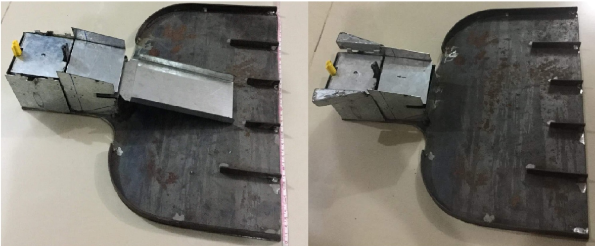
Dispositivo clasificador de huevos con bandeja de deslizamiento -imagen izquierda, sin bandeja de deslizamiento y con aditamentos en la esclusa de pesaje para alojar el emisor y sensor láser -imagen derecha (0)
