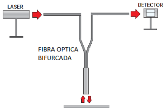
Figura 4. Esquema sensor óptico
